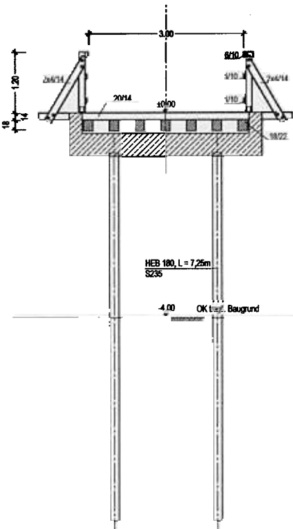
Querschnitt M 1:50
